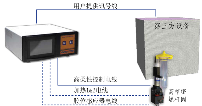
图3：高精度螺杆阀整合到第三方设备上
